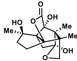
(+/-)-illisimonin A
