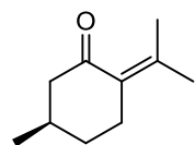
( R )-pulegone
