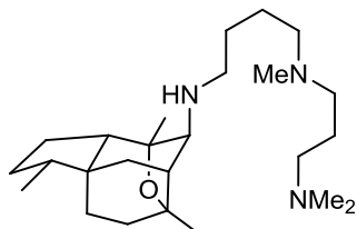
(-)-hispidospermidine
